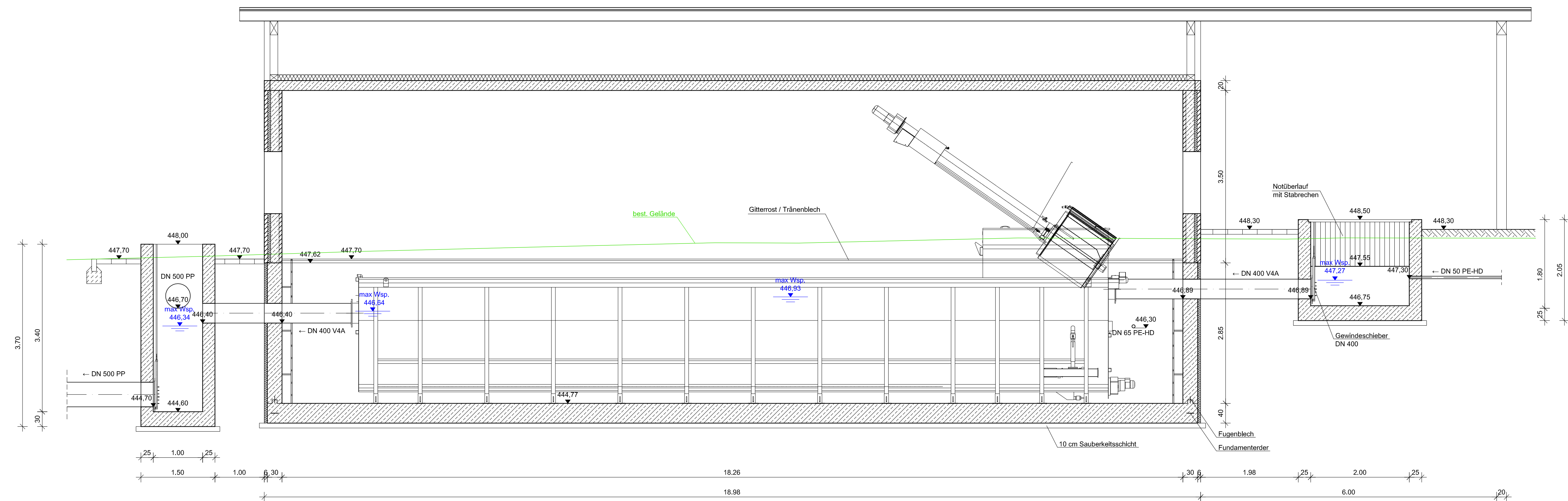
Schnitt A - A
