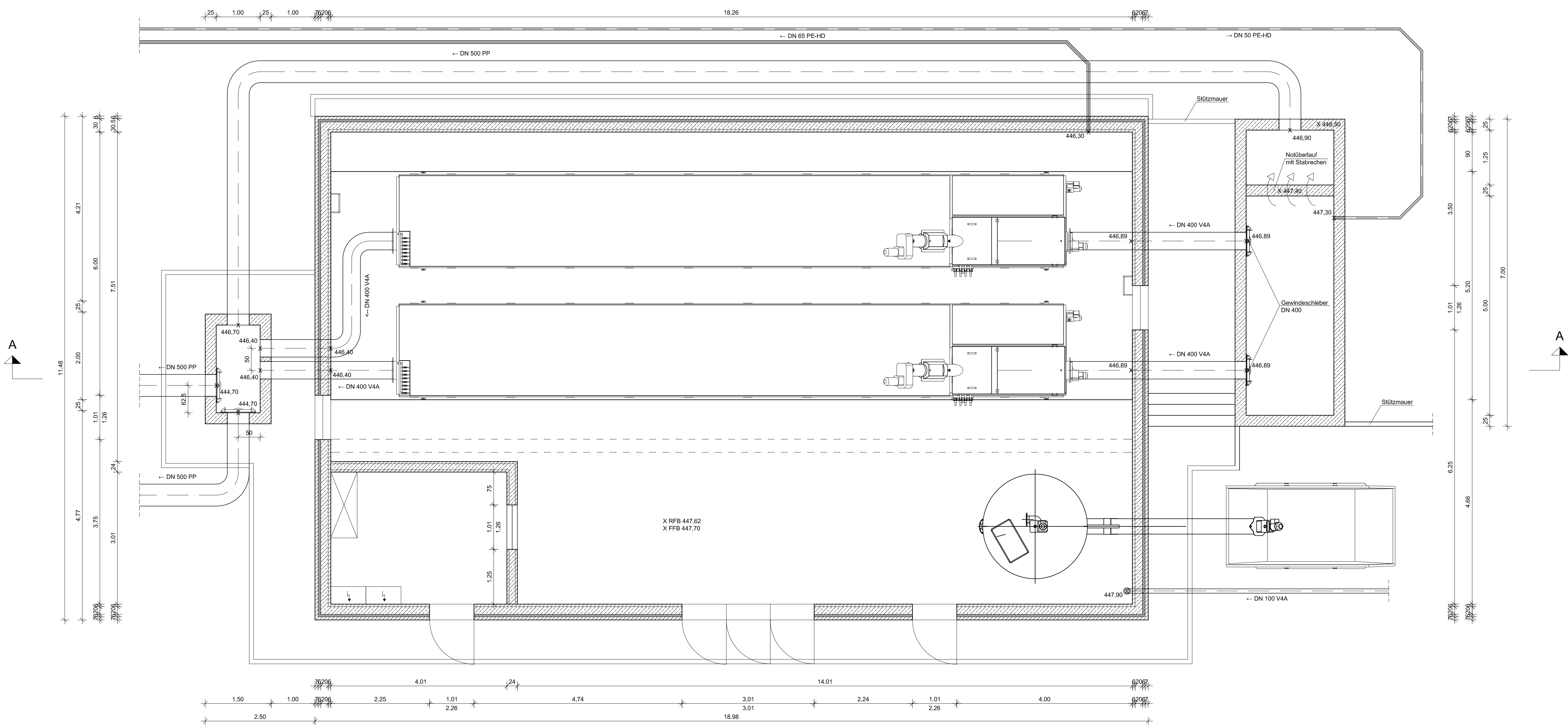
Draufsicht
