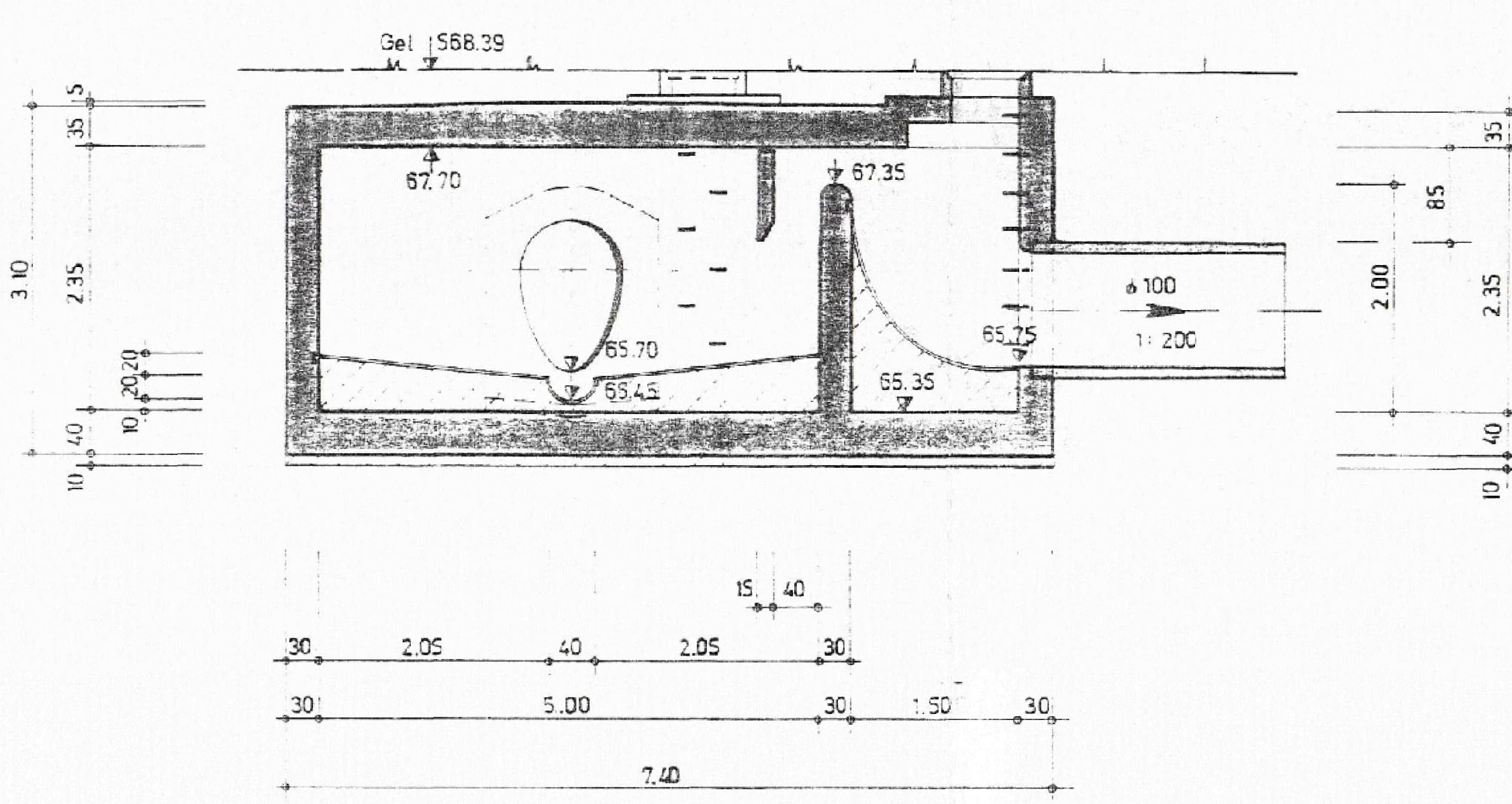
Schnitt B-B
