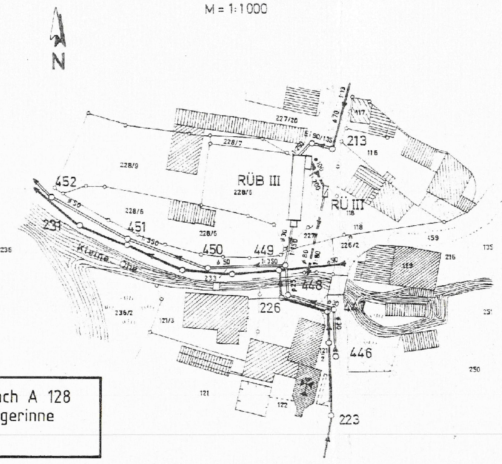
LAGEPLAN
