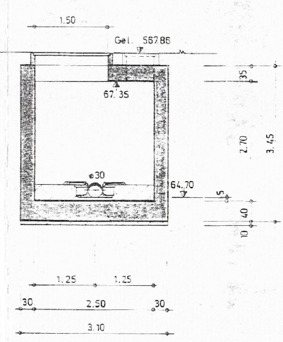
Schnitt C-C
